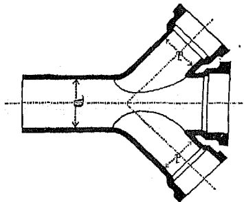
б) тройники.
