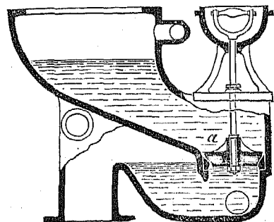
Черт. 29.
