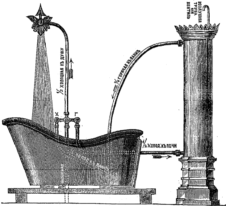
Чер. 69.
