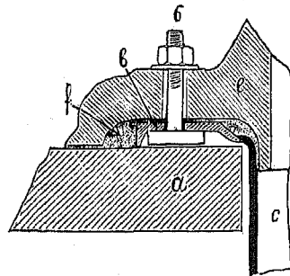
Чер. 144.
