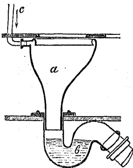
Чер. 30.
