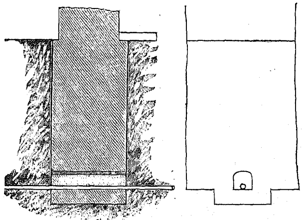
Чер. 135.
