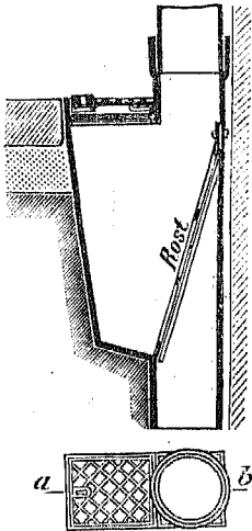
Чер. 107.
