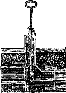
Чер. 119.
