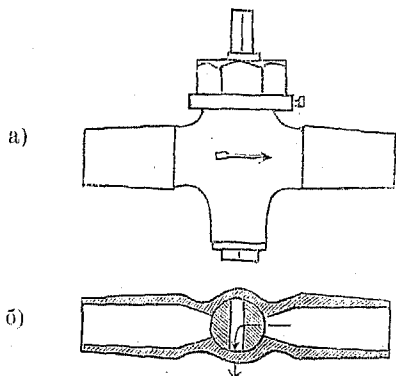
Черт. 88.
