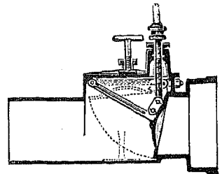
Чер. 118.
