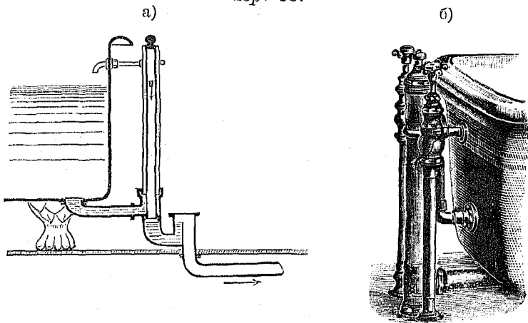
Чер. 68.
