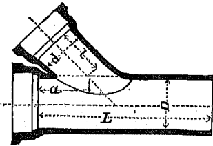
а) двойники.
