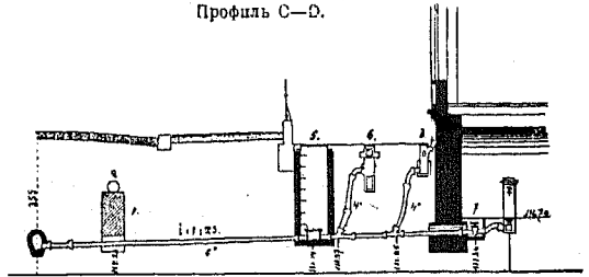
Профиль С—Д.
