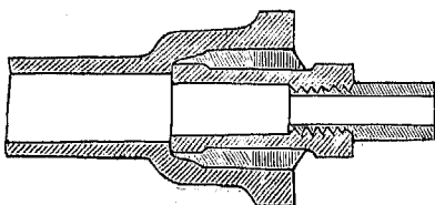
Чер. 137.
