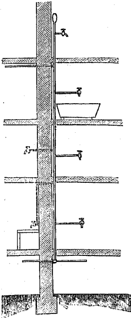
Чер. 122.
